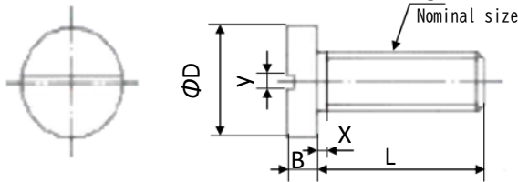
■ネジ Screw すりわり付 Slotted head 標準呼び Nominal size
