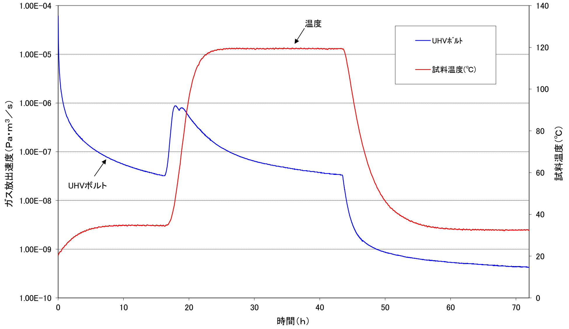
超高真空用ボルト ガス放出速度グラフ
