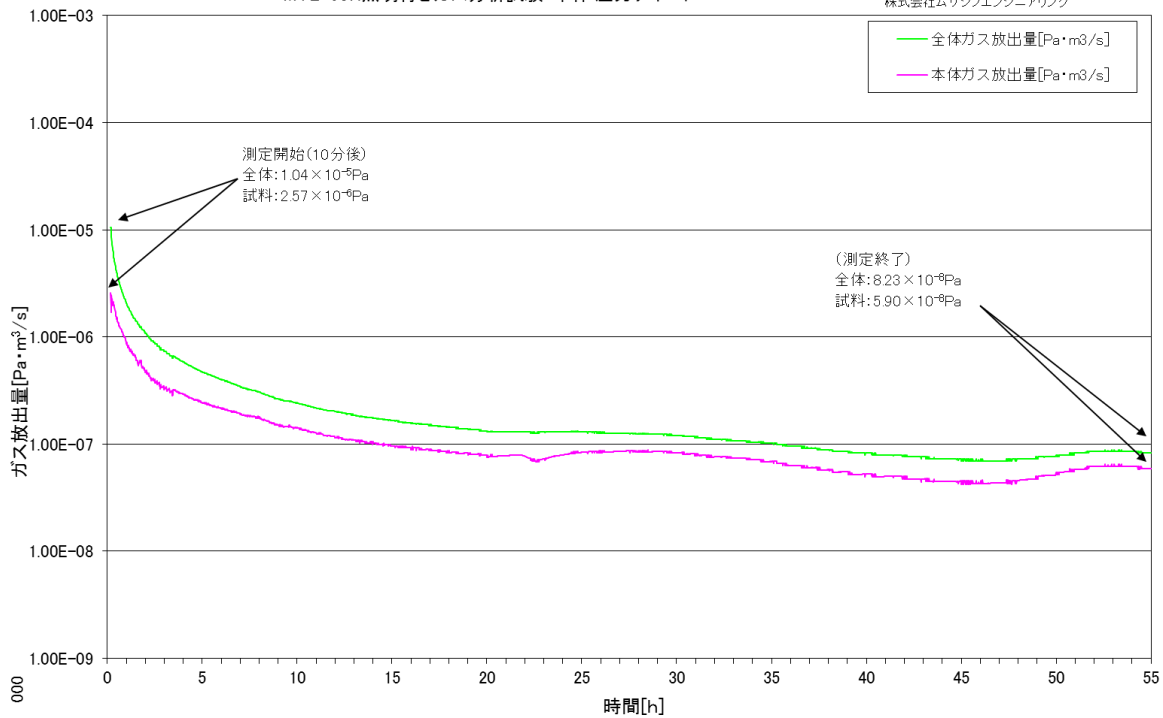
MVE-05H照明付きガス分析試験・本体 圧力チャート
