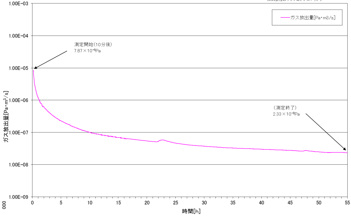
MVE-05H照明付きガス分析試験・空データ試験 圧力チャート
